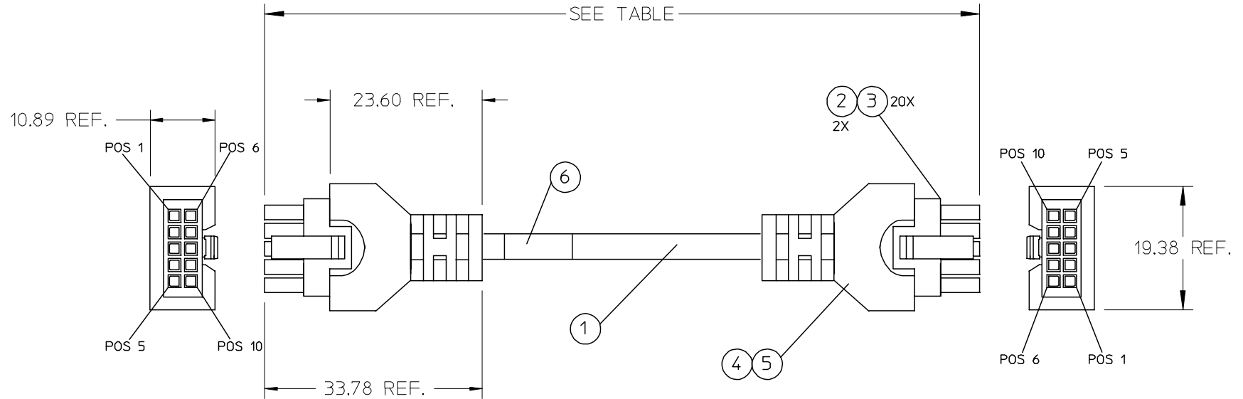
WIRING CHART
