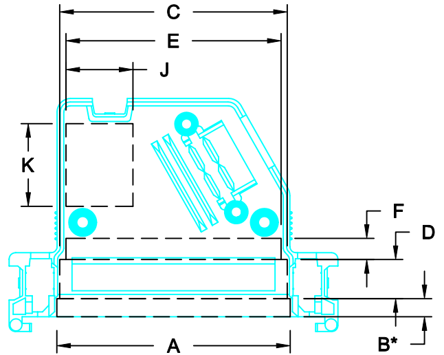
25-PIN
